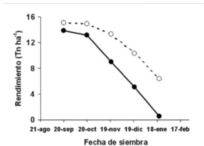
Figura 9: Rendimiento de maíz en función de la fecha de siembra en Pergamino (33°58`S; círculos blancos) y en Balcarce (37°45`S; círculos negros) para cultivos creciendo sin limitaciones hídricas, nutricionales ni sanitarias con densidad de 9 pl m -2 (adaptado de Cirilo 1994 y Cirilo, 2001)
