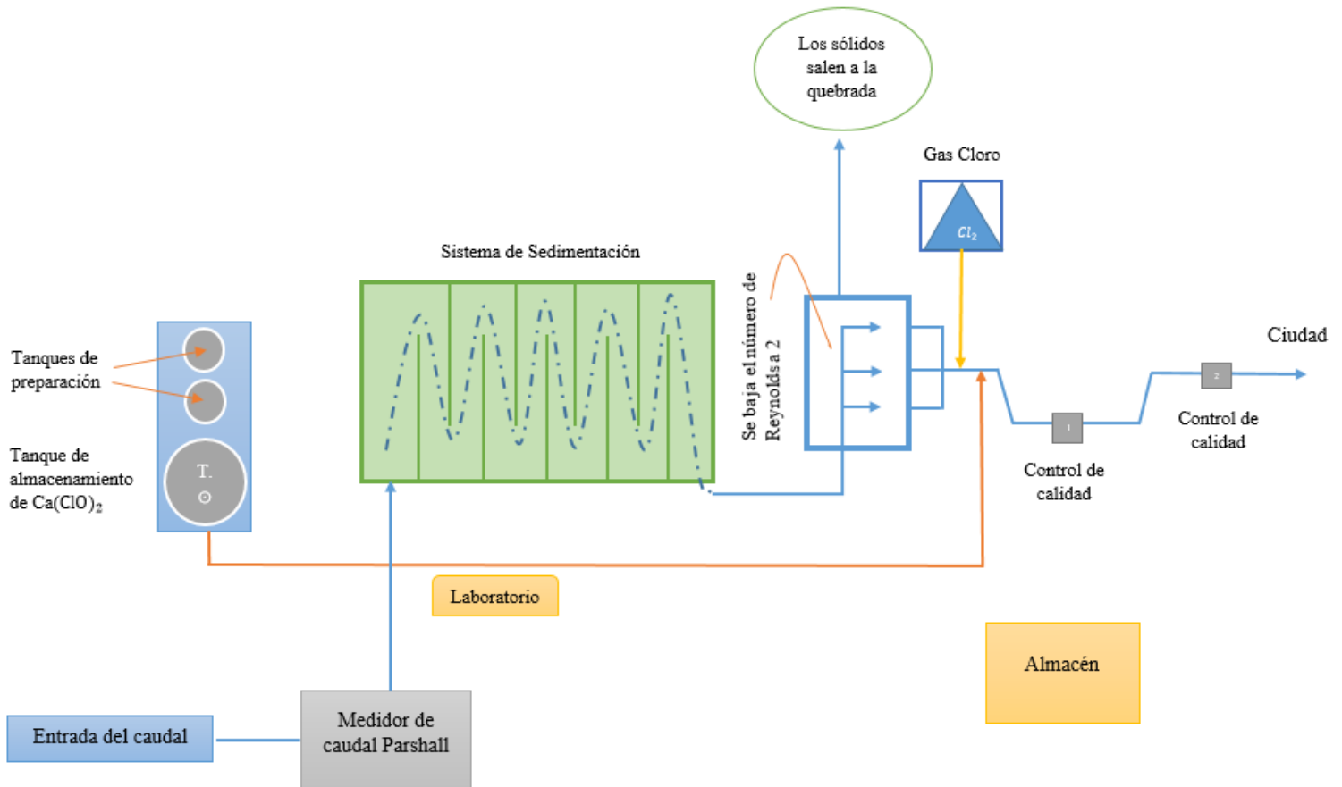
DIAGRAMA DE LA PLANTA DE CLORACIÓN DE TARIJA
