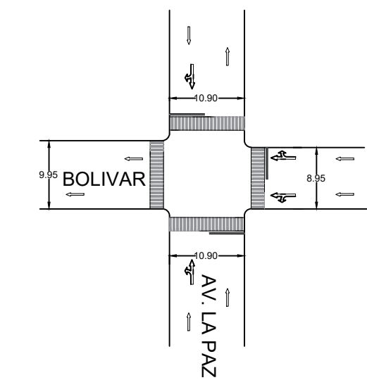
SEÑALIZACION EN INTERSECCION
