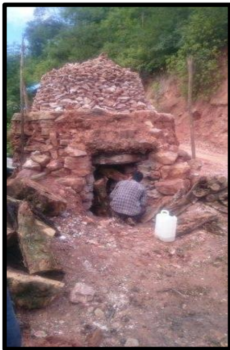
Horno Tipo Volcán Fuego Directo (Cantón Huayco, productor Sr. Mario Núñez).
