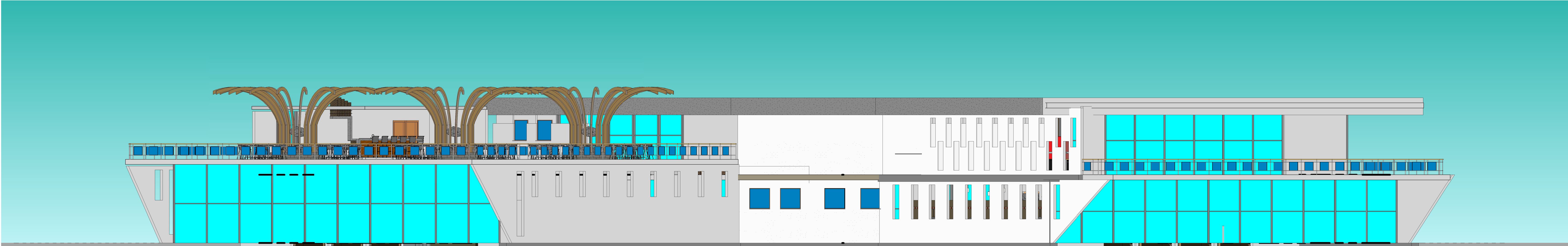
FACHADA POSTERIOR ESC 1 / 100
